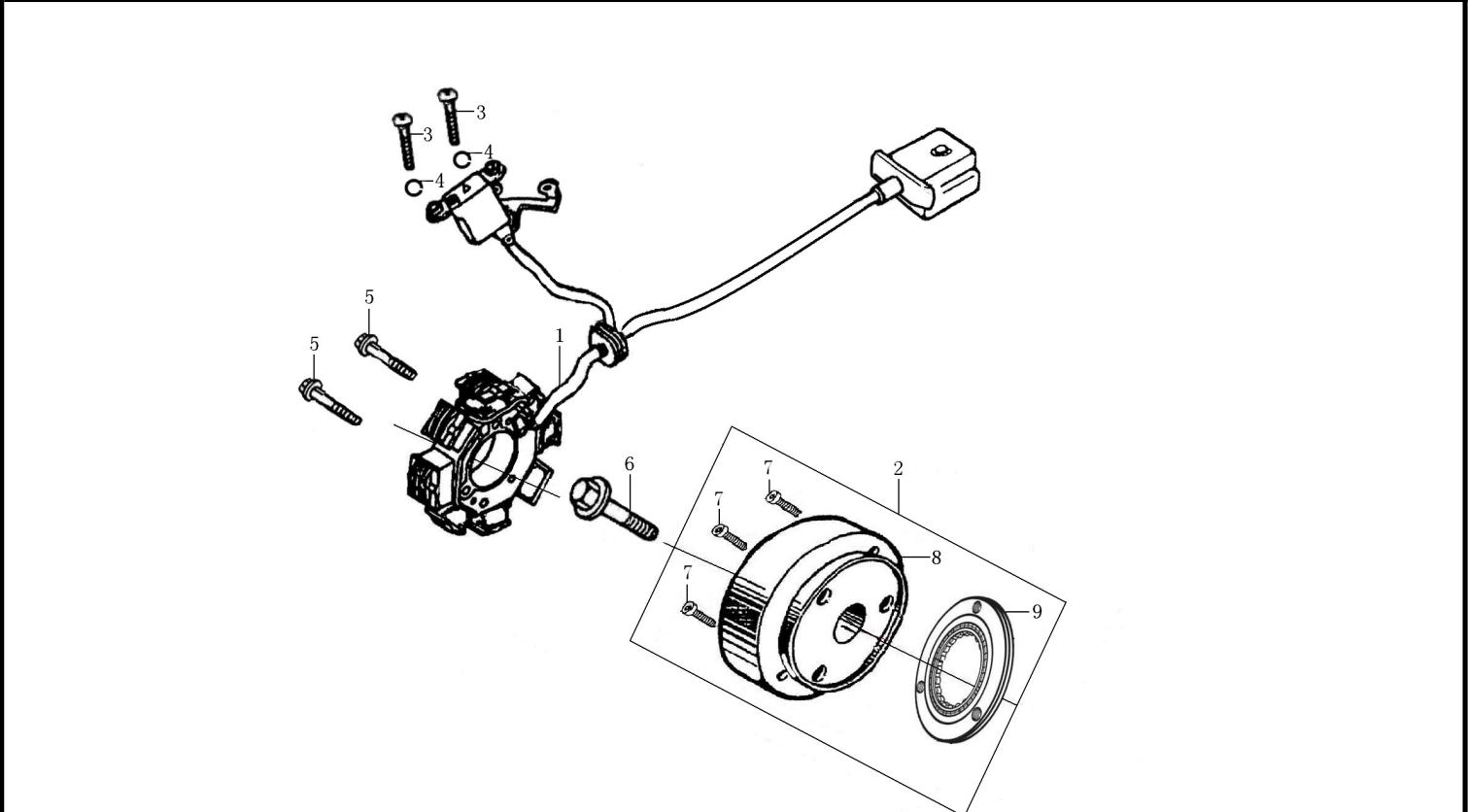
磁电机总成 MAGNETO COMP
