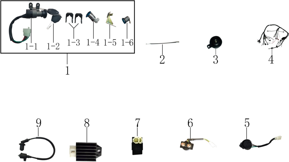
图5 电门锁、主电缆及全套电器件 switch,main cable&whole electric parts Ignit
