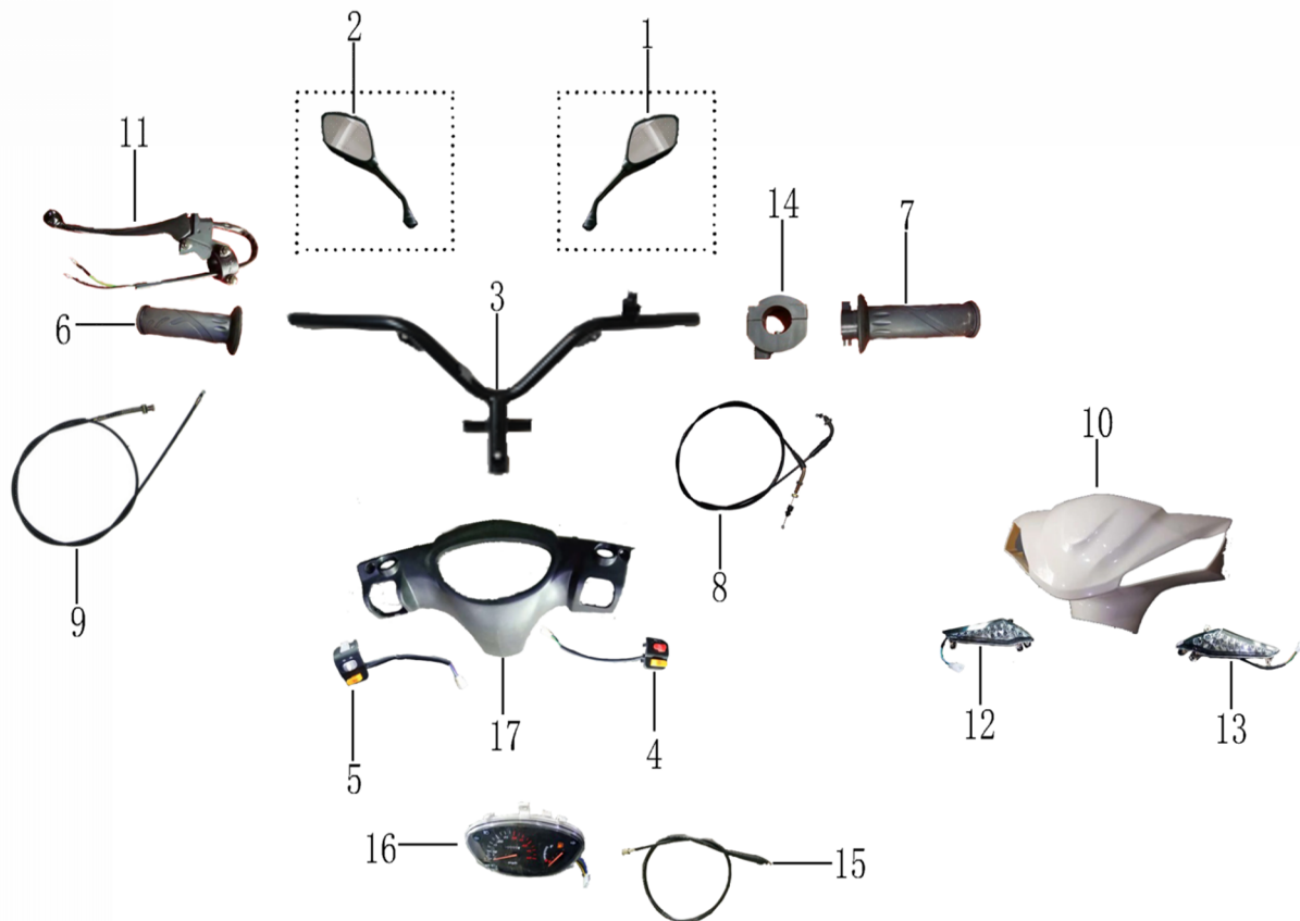
图1后视镜、方向把、头罩前后部及仪表总成、前左右转向灯
